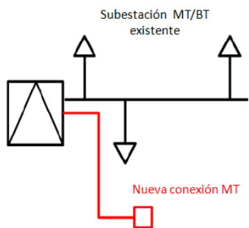
Figura 8 Conexión radial desde una subestación primaria.
