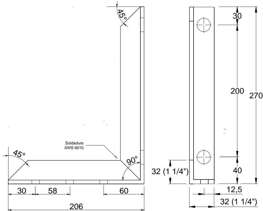
FIGURA 1 Herraje para Soporte de Seccionador de B.T. de 160 A.
