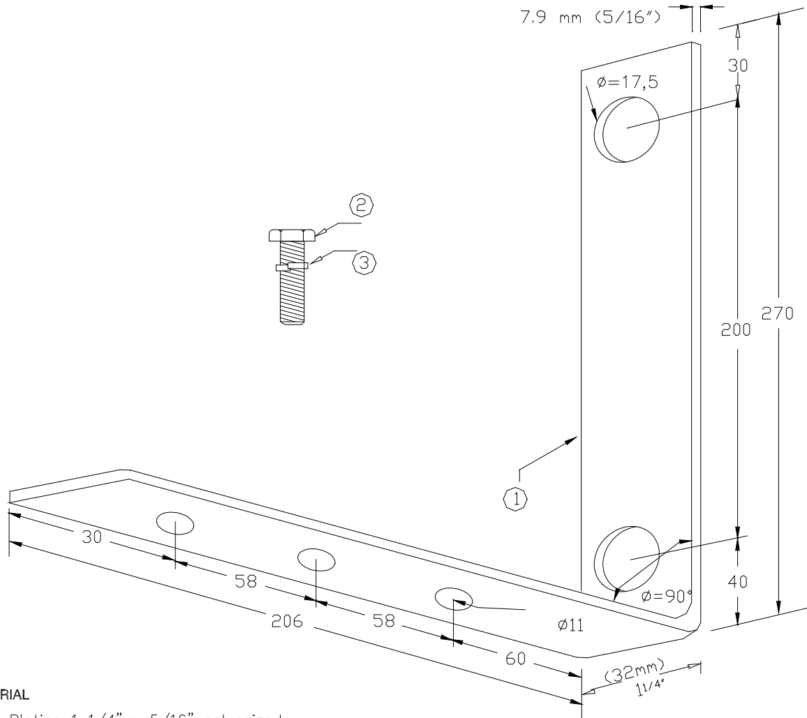
FIGURA 2 Herraje para Soporte de Seccionador de B.T. de 160 A. (Alternativa 1, con previa autorización de CODENSA S.A.)
