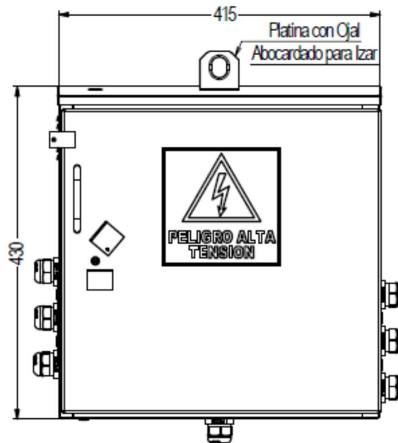
FIGURA 2. VISTA FRONTAL
