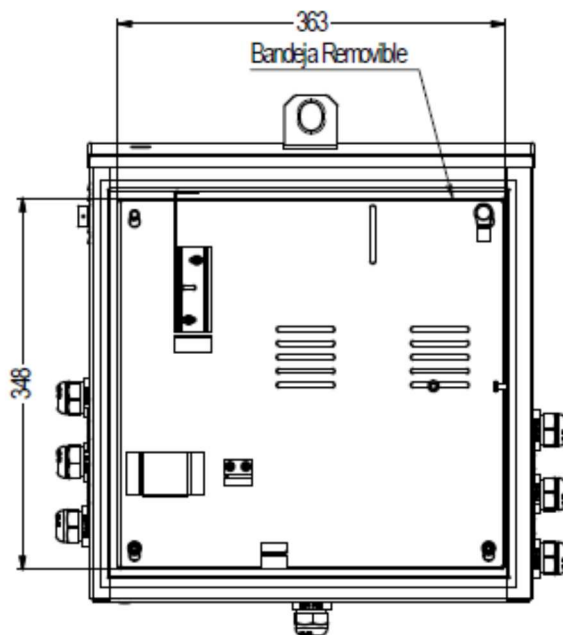
FIGURA 1. VISTA INTERIOR
