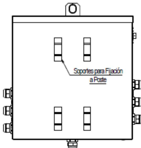
FIGURA 5. VISTA POSTERIOR
