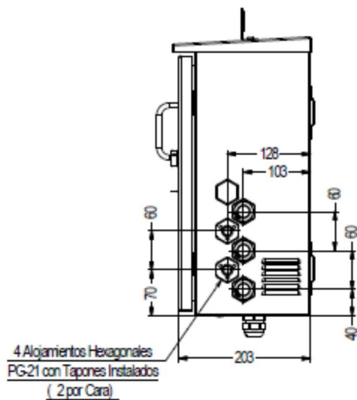
FIGURA 3. VISTA LATERAL
