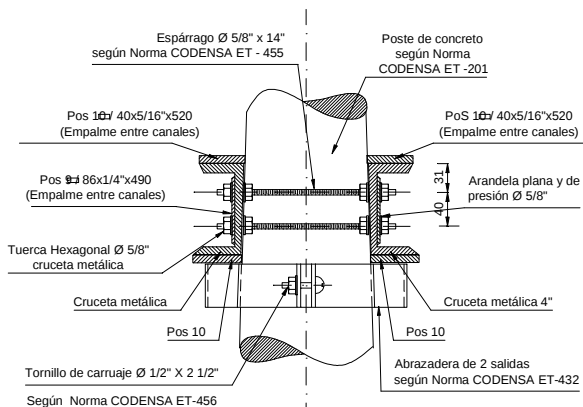
VISTA B-B'
