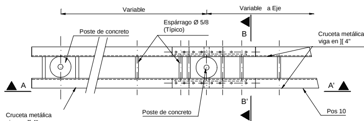
PLANTA TÍPICA DE CRUCETAS
