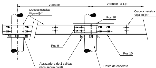
VISTA A - A'
