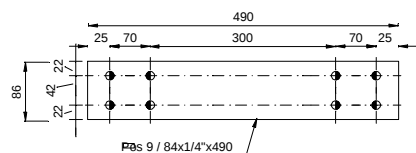
VISTA A - A'
