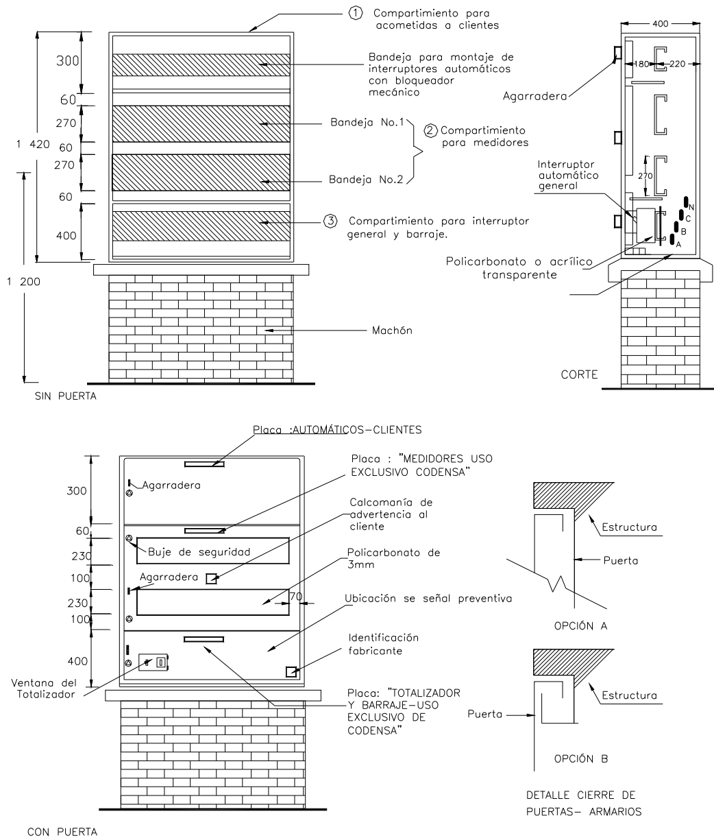
FIGURA 1 - ARMARIO DE MEDIDORES DE 6 A 10 CUENTAS TRIFASICAS ACOMETIDA POR DEBAJO Y PARCIALES POR DEBAJO
