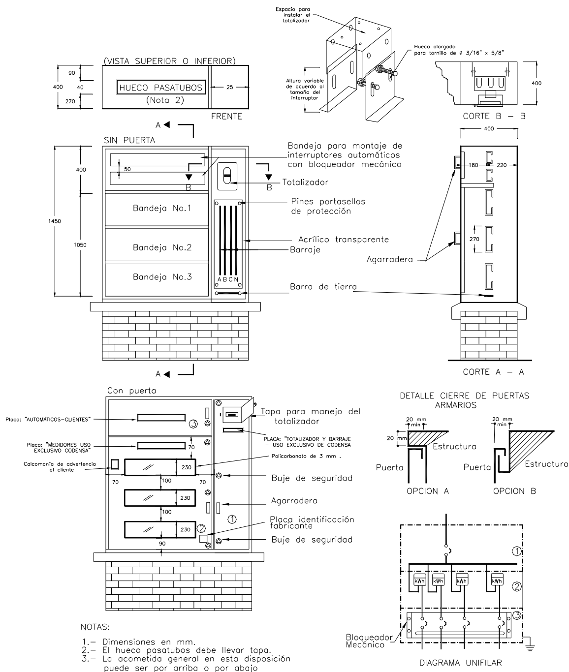
FIGURA 5 - ARMARIO CON TOTALIZADOR Y BARRAJE LATERAL
