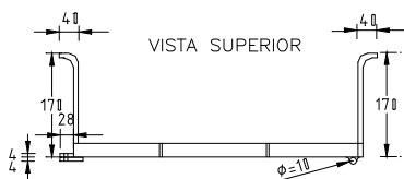
PUERTA
