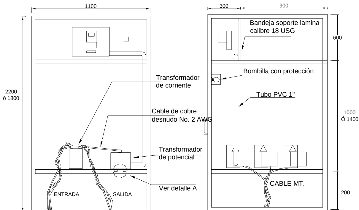
VISTA FRONTAL SIN PUERTA
