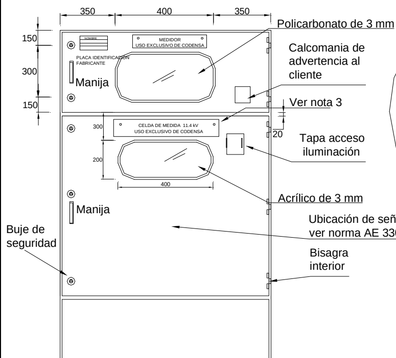
VISTA FRONTAL CON PUERTA
