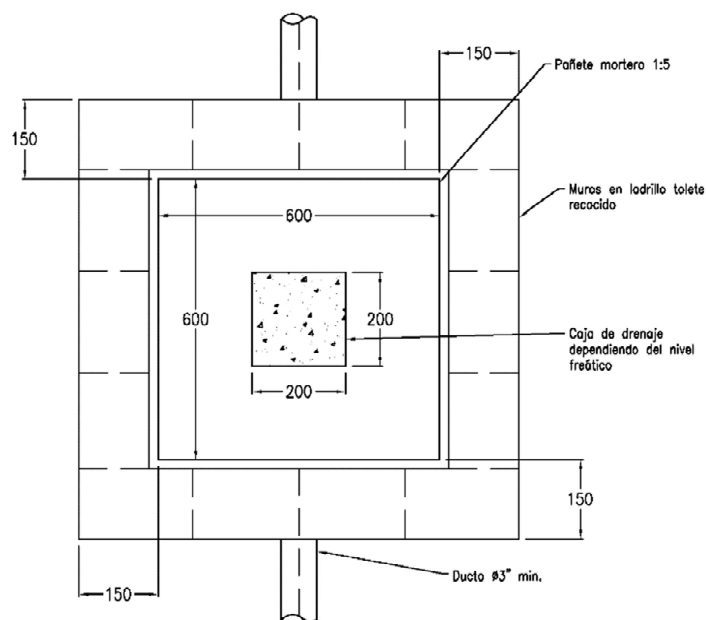
PLANTA CAJA Y MUROS
