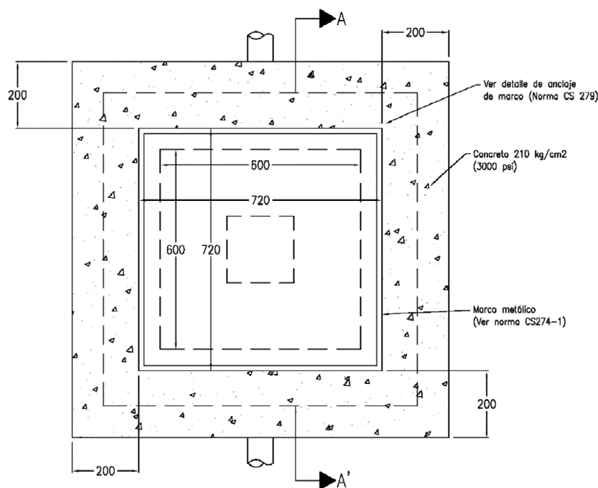
PLANTA CAJA CON MARCO
