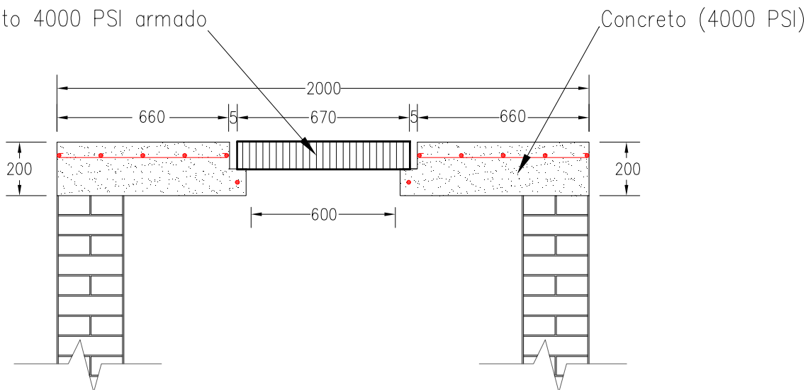
DETALLE HIERROS CORTE CORTE B-B'
