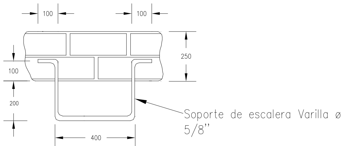
DETALLE SOPORTE PARA ESCALERA
