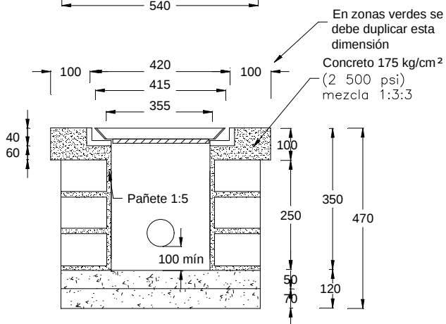
CORTE A-A'
