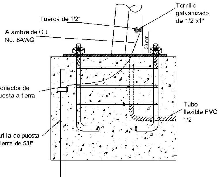
DETALLE DE LA BASE Y DE LA PUESTA A TIERRA
