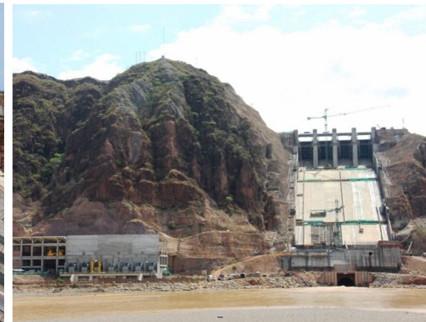
Panorámica de la Estructura de Control Aguas Abajo del vertedero
