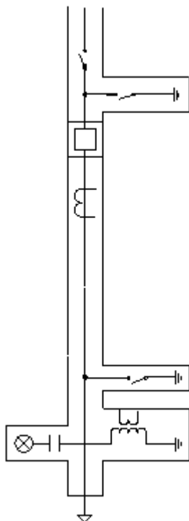
Celda Transformador
