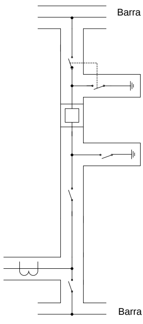
Celda Transformador
